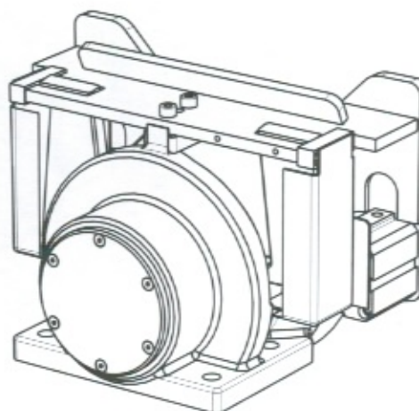
STO A50 chuck without shaft end
