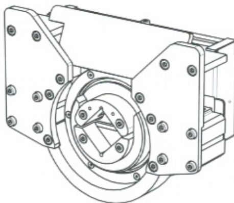
Boschert-Chuck A50
