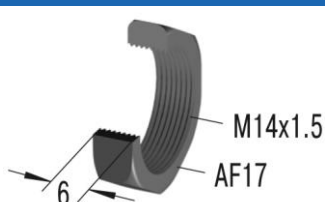
Przeciwnakrętka KM14
