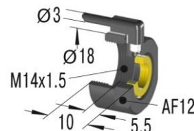
Tuleja zderzaka z czujnikiem AS14
