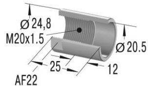
Tuleja zderzaka AH20-V4A
