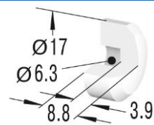
Głowica nylonowa PP225
