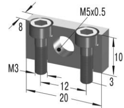
Kołnierz zaciskowy MB5SC2
