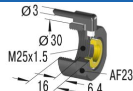
Tuleja zderzaka z czujnikiem AS25
