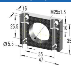
Kołnierz uniwersalny UM25
