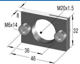
Kołnier prostokątny RF20
