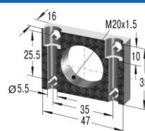
Kołnier uniwersalny UM20
