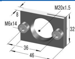
Kołnier prostokątny RF20
