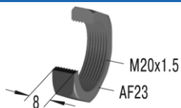
Przeciwnakrętka KM20
