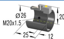
Kołnier uniwersalny UM20
