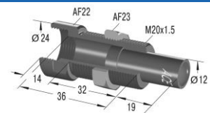
Głowica stalowa PS20
