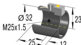
Kołnierz uniwersalny UM25
